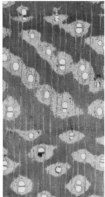
Coupe transversale (× 14)
